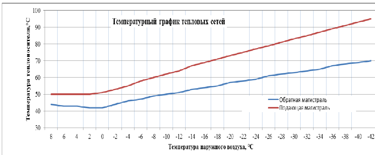
Рисунок 2 – Температурный график котельных
