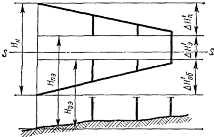
Рисунок 8 Пьезометрический график тепловой сети при пропорциональной разрегулировке абонентов.
